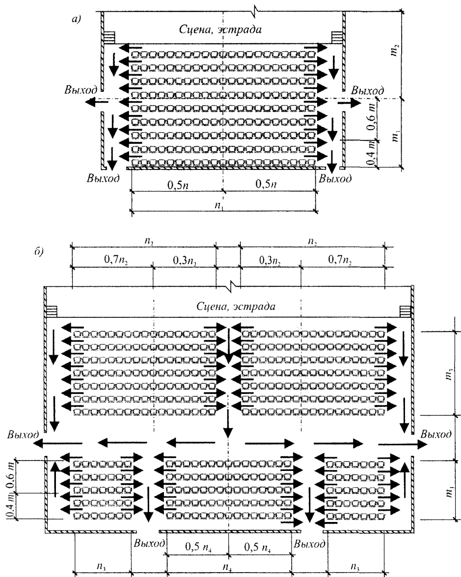
а - с боковыми (продольными) проходами; б - с поперечным проходом
