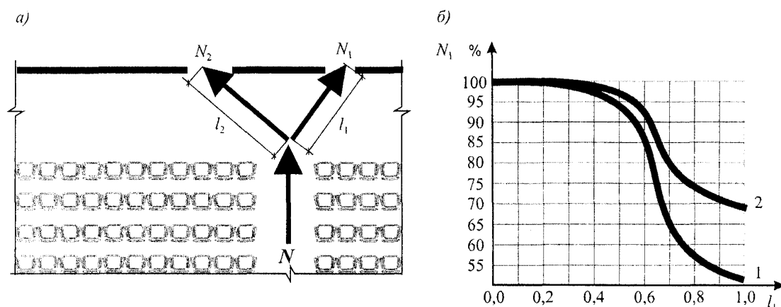
а - схема распределения потока численностью N , чел.; б - влияние соотношения между расстояниями до выходов на распределение численности людей из общего потока, направляющихся: 1 - к ближайшему из двух одинаковых выходов l_1 : наружу, в лестничные клетки, на открытые лестницы; 2 - к открытой лестнице l_1 или в лестничную клетку l_2
